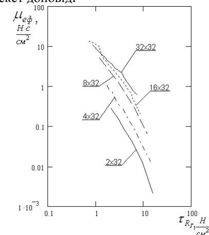
Рис. 2. Залежності ефективного в'язкості від напруження зсуву під час течії полістиролу в прямокутних каналах
