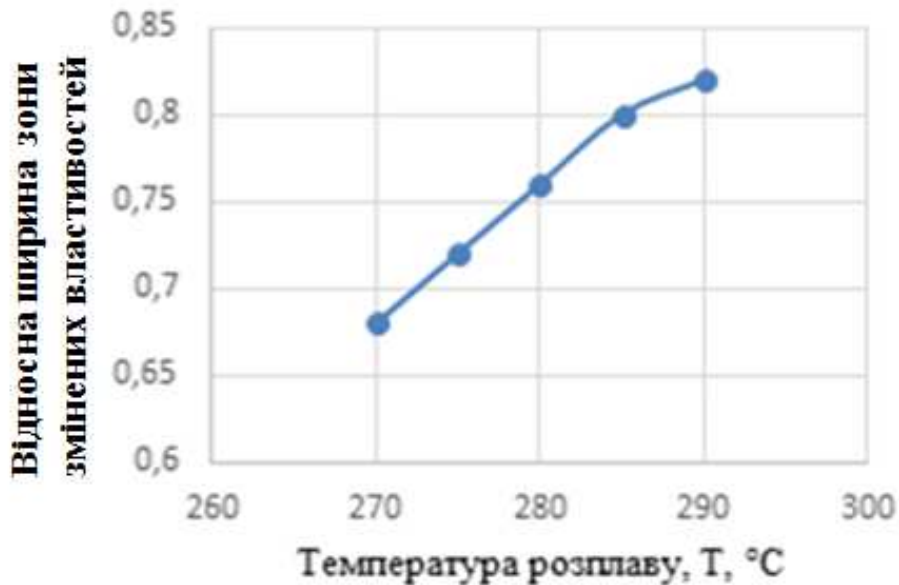
Рисунок 5.2 – Графік залежності відносної ширини зони змінених властивостей від температури лиття
