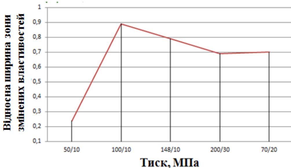
Рисунок 5. 5– Графік залежності ширини зони змінених властивостей від зміни тиску, при вихідних даних: температура форми = 90 С, час= 0,53 с, Температура розплаву: від 275 до 290С
