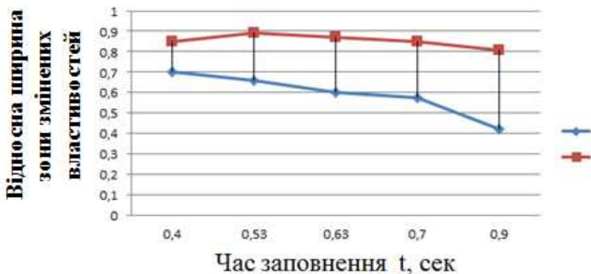
Рисунок 5. 4– Графік залежності ширини зони змінених властивостей від часу заповнення при вихідних даних:
